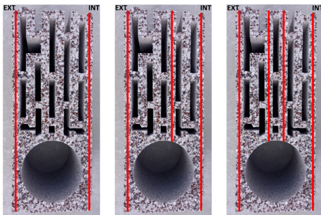
Figure 13 – Répartition des cordons de colle sur les blocs d'angle (granulats légers)
