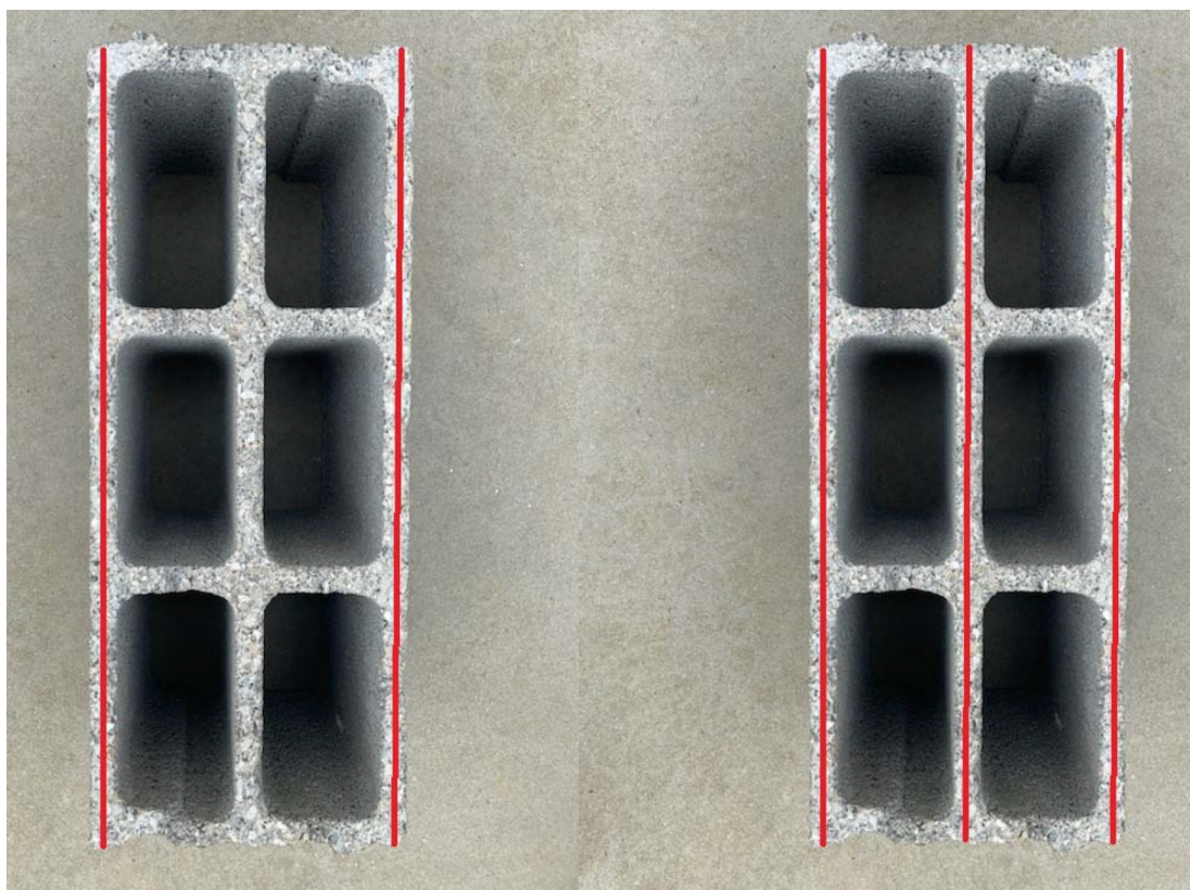
Figure 10 – Répartition des cordons de colle sur les blocs standards (granulats courants)
